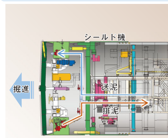
泥水式シールド工法模式図
